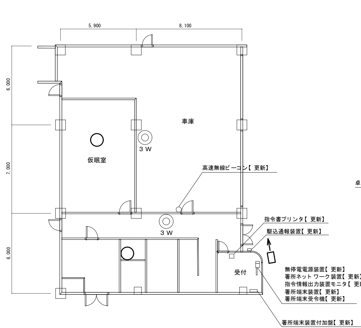
吹上分署 1 階 平面図
