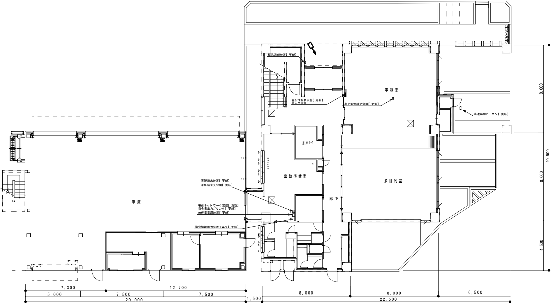
天神分署 1 階 平面図
