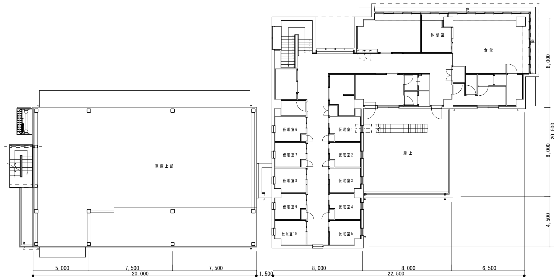
天神分署 2階 平面図
